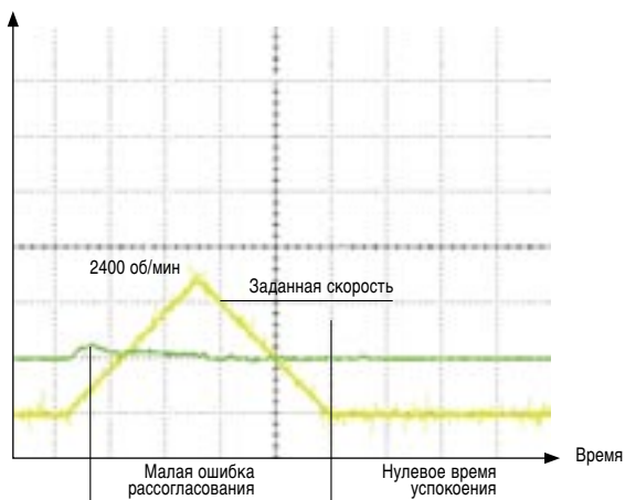
Привод XtraDrive
