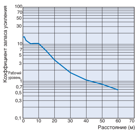
E3Z-T61/T81 (Инфракрасное излучение)
