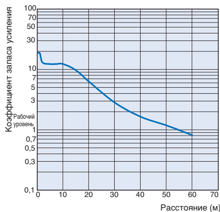
E3Z-T61/T81 (Красный свет)
